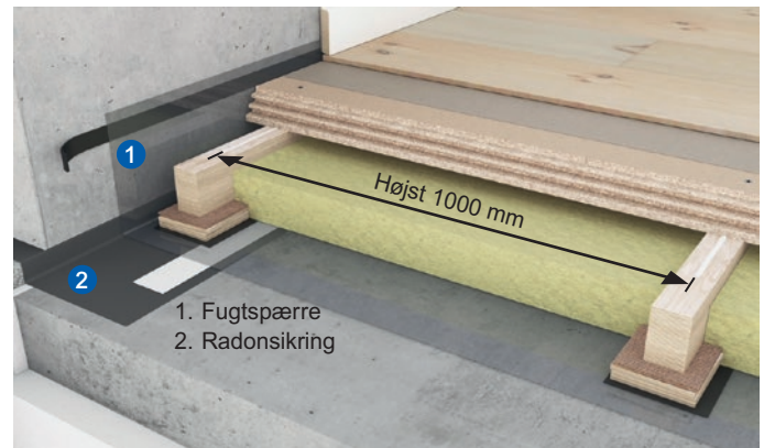
Figur 1 Undergulve på terrændæk bør altid udføres med en fugtspærre og radonsikring på betonoverfladen.
