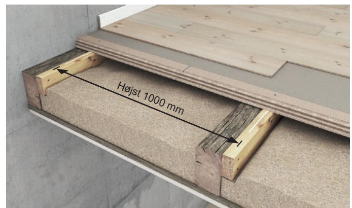
Figur 2 Ældre etagedæk oprettet med planker. Ved store spænd kan der monteres planker på begge sider af gulvbjælkerne for at reducere spændvidden.
